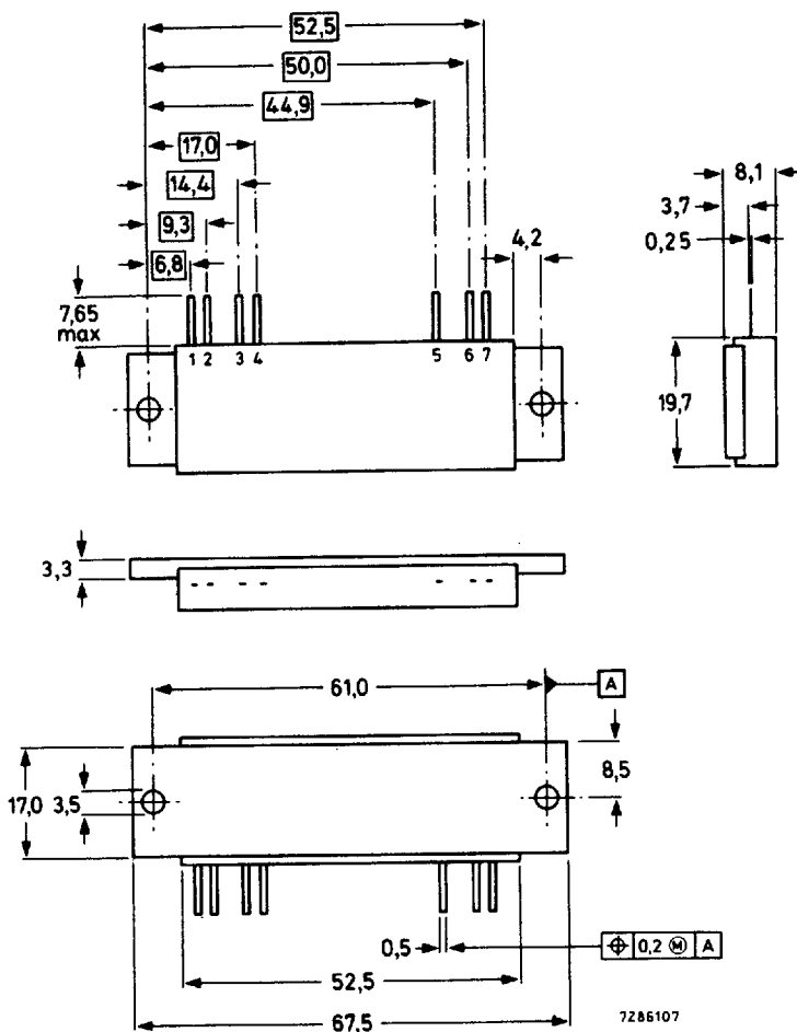
Fig. 1 SOT132B.
