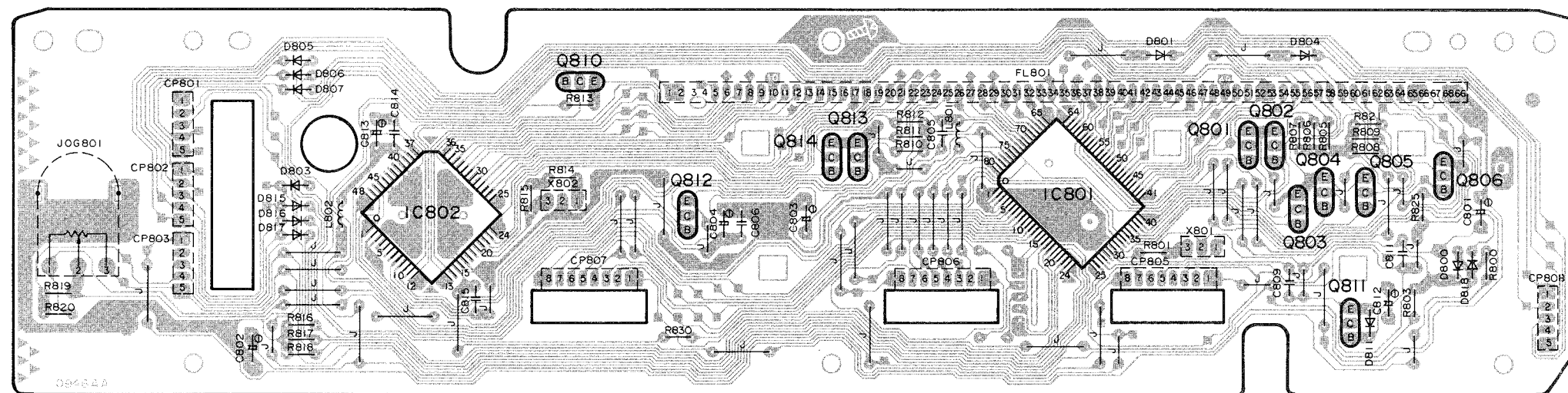
A FL P.C.B. (REP1460A-S)
