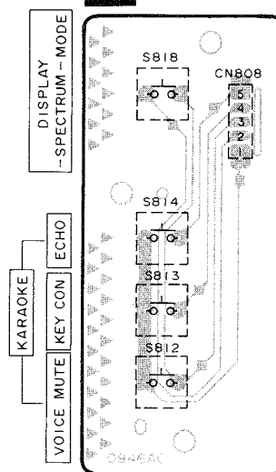
B KARAOKE P.C.B. (REP1460A-S)
