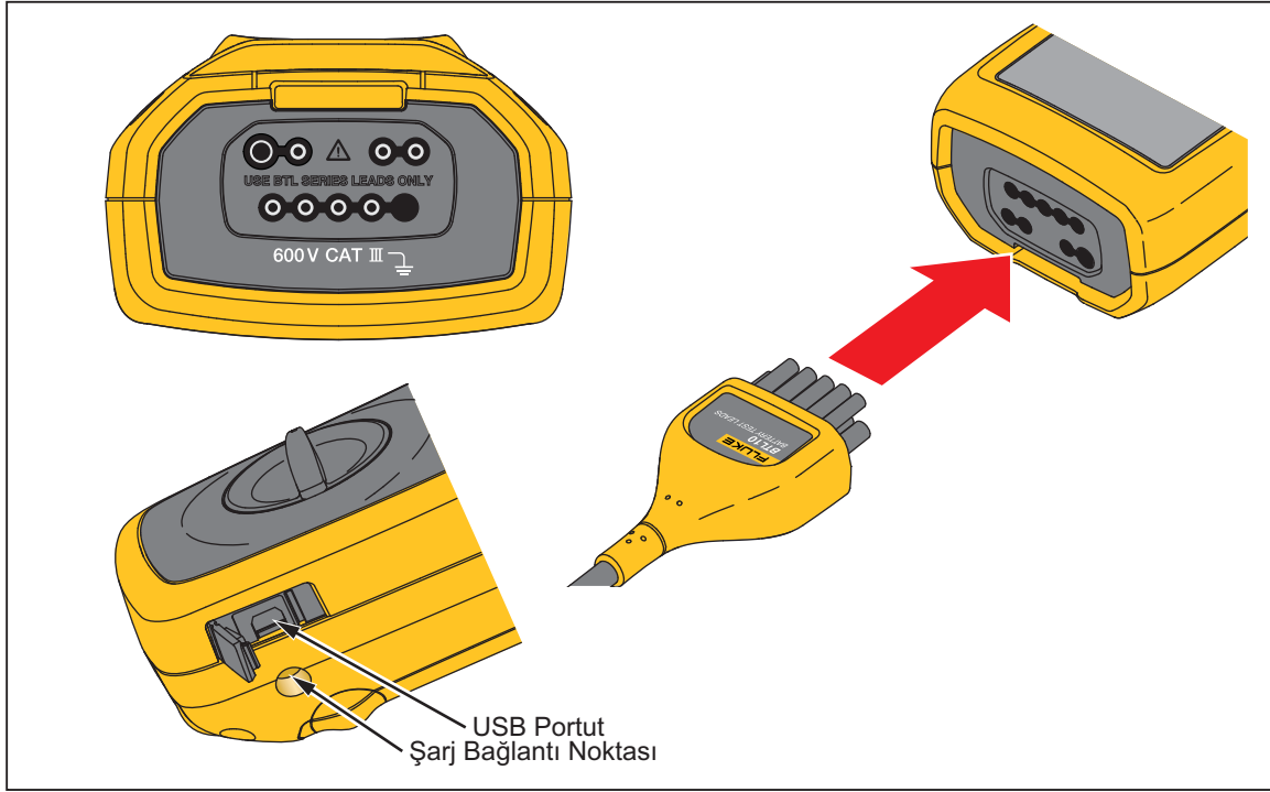
Şekil 1-2. G/Ç Terminalleri
